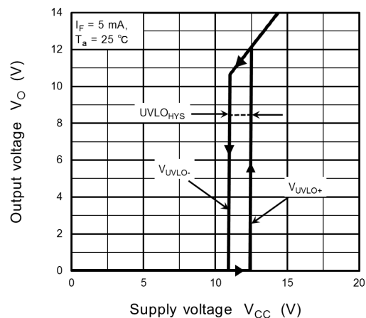
Fig. 13.2.6 V_O(V_{UVLO}) - V_{CC}
